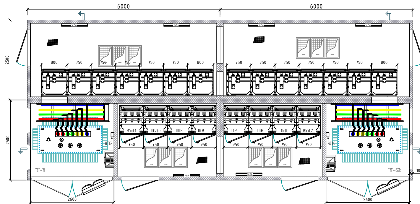
Пример компоновочного решения для ЗКТПу до 1600-2000-2500кВА напряжением 6(10)/0,4кВ
